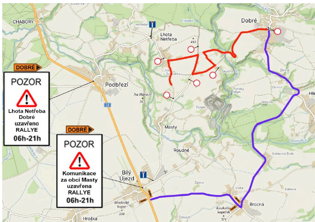
Situační schéma s vyznačeným umístěním přechodného dopravního značení
